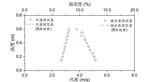
图 6 风洞试验模拟的风速和湍流度剖面
