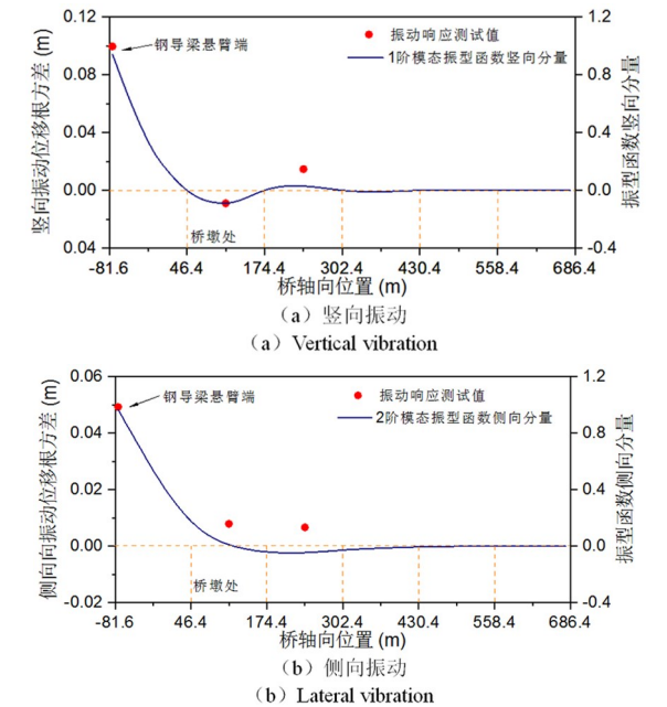
图 7 桥轴线不同测点处桥梁振动位移均方差( V=40.5\text{ m/s} )
