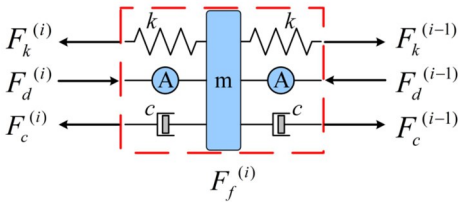
图 2 单元受力分析示意图
