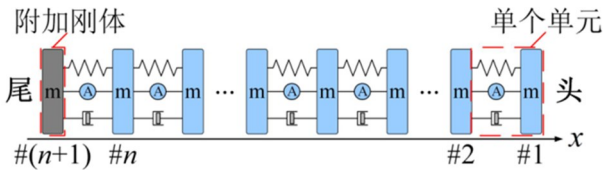
图 1 多单元仿蠕虫机器人力学模型简图
