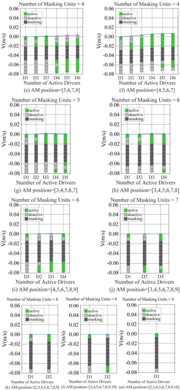
图9 施加动作掩蔽后不同驱动器个数对应的最优排布
