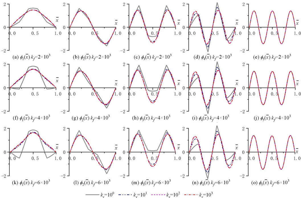
图 3 典型 k_f 和 k_r 组合下浮桥结构前 5 阶模态图
