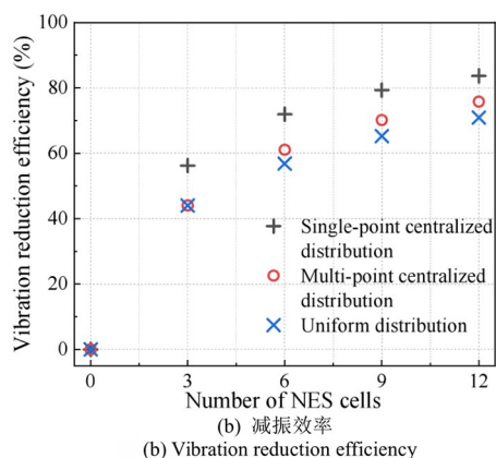
图 9 不同 NES 安装方式下系统的幅频响应曲线与减振效率(二阶固有频率附近)
