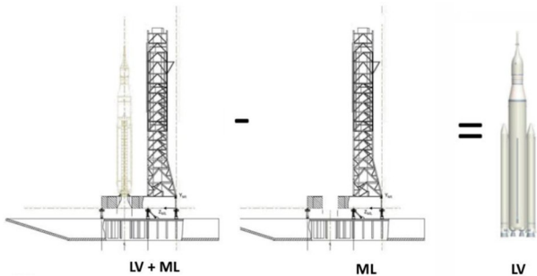
图1 SLS的加速度解耦方法示意 Fig.1 Conceptual acceleration decoupling
