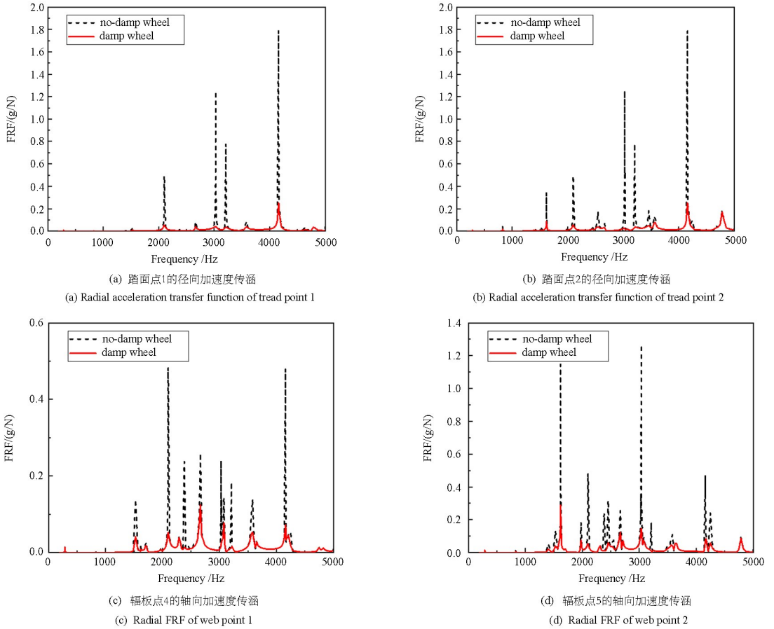
图 7 有无阻尼器车轮振动频响函数
