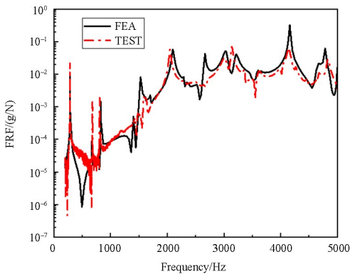
图9 踏面点1的径向加速度传递函数仿真与实验结果
