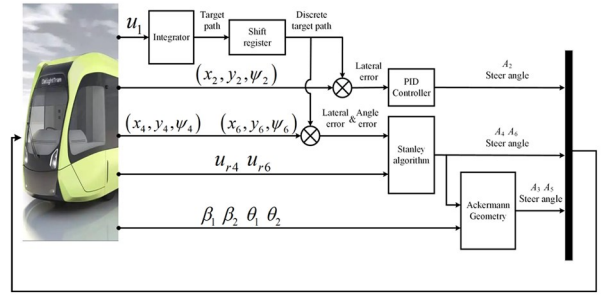
图 4 控制方法流程图
