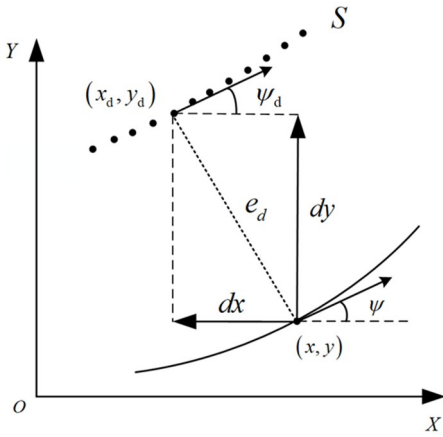
图 5 横向偏差示意图 Fig. 5 Lateral error diagram
