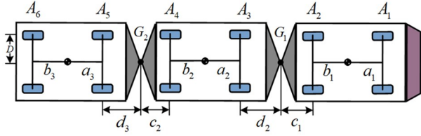
图 2 虚拟轨道列车结构图
