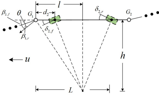
图 7 基于单轨线模型的车轮转向
