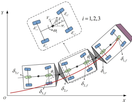
图 3 单轨线模型示意图
