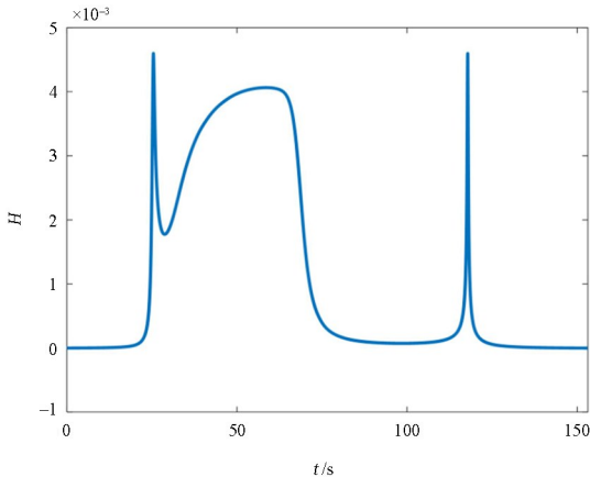
图7 哈密顿函数曲线 Fig. 7 Hamiltonian function
