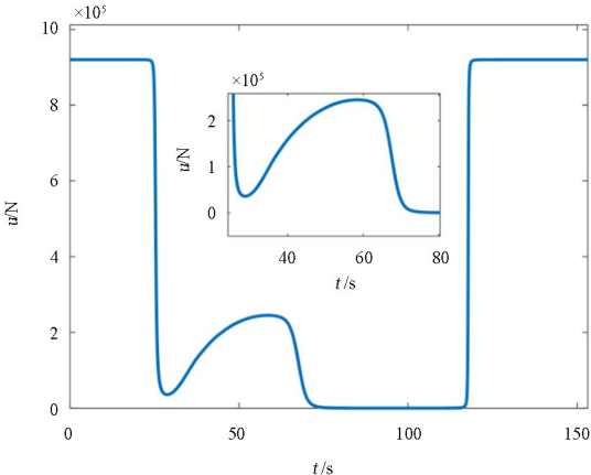
图4 推力曲线 Fig. 4 The thrust curve
