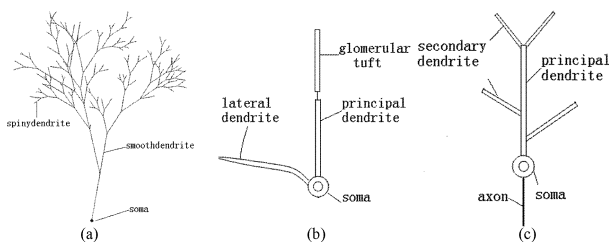
图1 三类主神经元几何形态,(a)浦肯野神经元,(b)僧帽神经元,(c)CA1 锥体神经元
