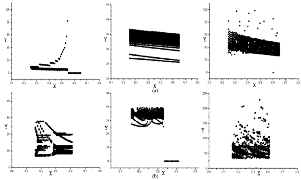
图5 (a)直流电刺激从0.25nA到0.65nA的变化过程中,三种主神经元:CA1锥体神经元、浦肯野神经元和僧帽神经元动作电位的ISI变化图,X轴为直流电刺激强度,Y轴为ISIs;(b)交流电刺激频率W从0.16到0.41的变化过程中,三种主神经元:CA1锥体神经元、浦肯野神经元和僧帽神经元动作电位的ISI变化图,X轴为交流电刺激频率,Y轴为ISIs
