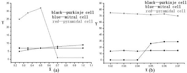
图4 (a)为在直流电刺激下,三类主神经元胞体动作电位的平均发放频率图,X轴为直流电刺激强度:0.25nA~1.0nA,Y轴为平均发放频率;(b)为在交流电刺激下,三类主神经元胞体动作电位的平均发放频率图,X轴为交流电刺激频率W:0.02~0.07,Y轴为平均发放频率
